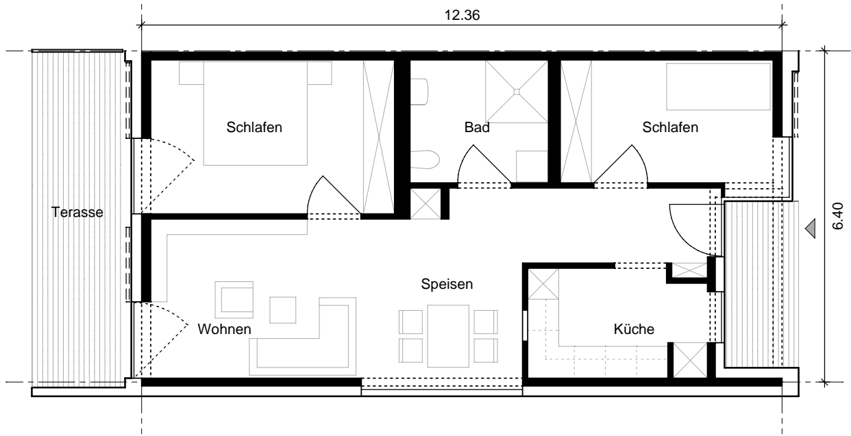
Wohnungstyp B
