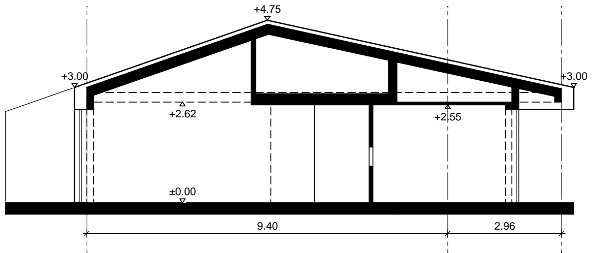
Prinzipschnitt
